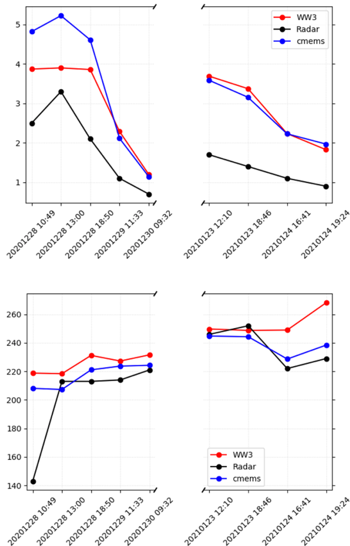
Figura 64 altezza d'onda in metri (pannello superiore) e direzione (pannello inferiore) per modello e radar
