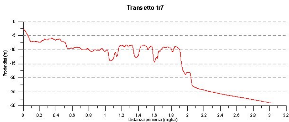
Fig. 83 Profilo batimetrico relativo al transetto “tr7”.
