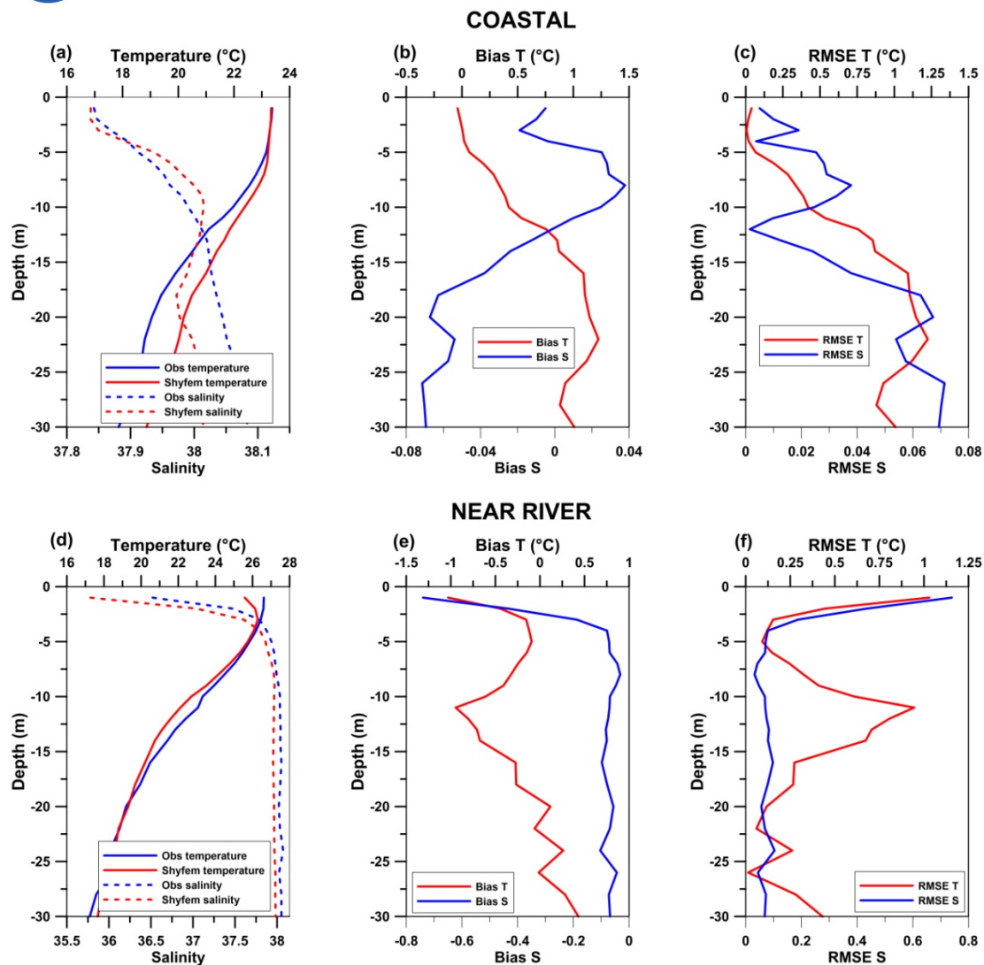
Fig. 57 validazione del modello attraverso la comparazione con i dati CTD "costieri" (a, b, c) e "fluviali" (d, e, f)
