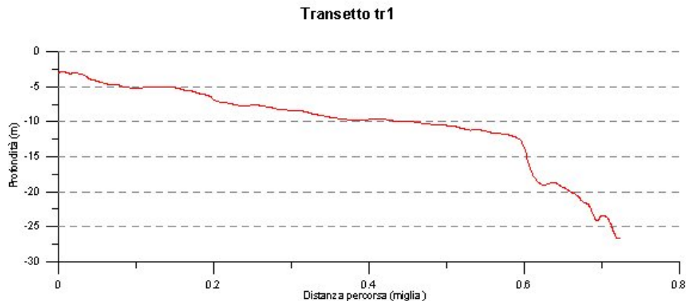
Fig. 82 Profilo batimetrico relativo al transetto "tr1".
