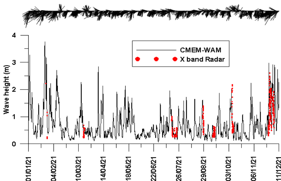
Fig 6: il grafico in basso mostra il confronto tra le altezze d'onda misurate dal radar (pallini rossi) e calcolate dal modello WAM di COPERNIUS (linea nera continua), l'immagine in alto rappresenta lo stick plot della direzione del moto ondoso analizzata dal modello.
