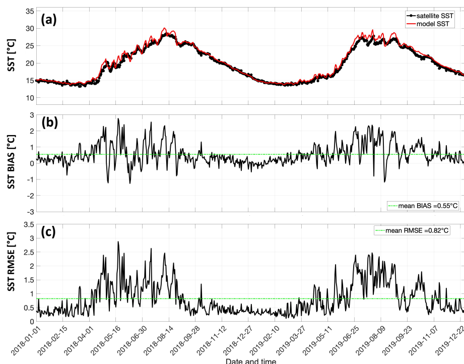
Fig. 55 Comparazione tra i dati temperatura media superficiale del modello e del satellite sull'intero dominio di calcolo (a). Vengono inoltre mostrate le metriche di bias (b) e RMSE (c).
