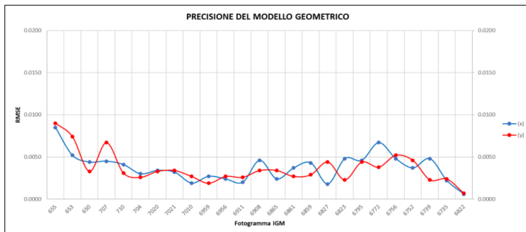
Fig. 71 Confronto della RMSE in X e in Y tra tutti i fotogrammi ortorettificati
