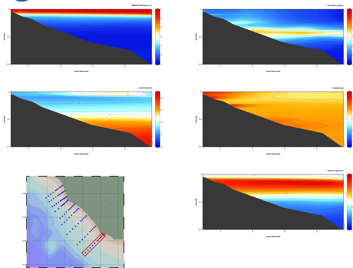
Fig.17 Campagna Estate 2020: sezione profondità distanza del transetto TR12 dell'andamento delle variabili temperatura, salinità, clorofilla, torbidità e ossigeno disciolto
