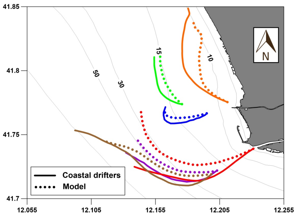
Fig. 60 Confronto tra le traiettorie delle boe lagrangiane (linee continue) e traiettorie simulate (linee tratteggiate).
