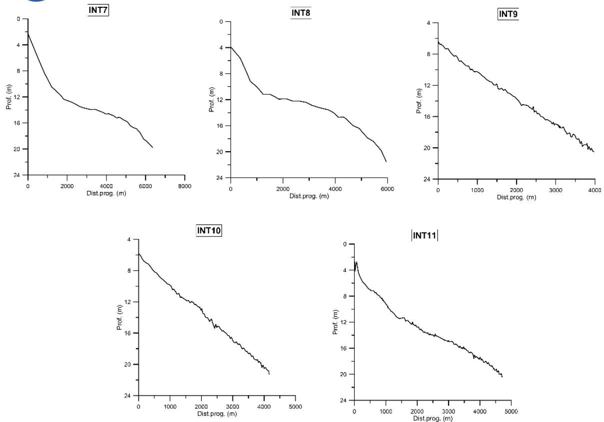
Fig. 26 Profili morfologici acquisiti durante le due campagne di misura
