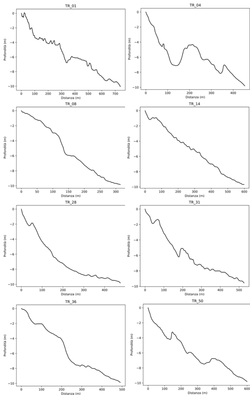
Figura 78 alcuni profili batimetrici della zona a nord
