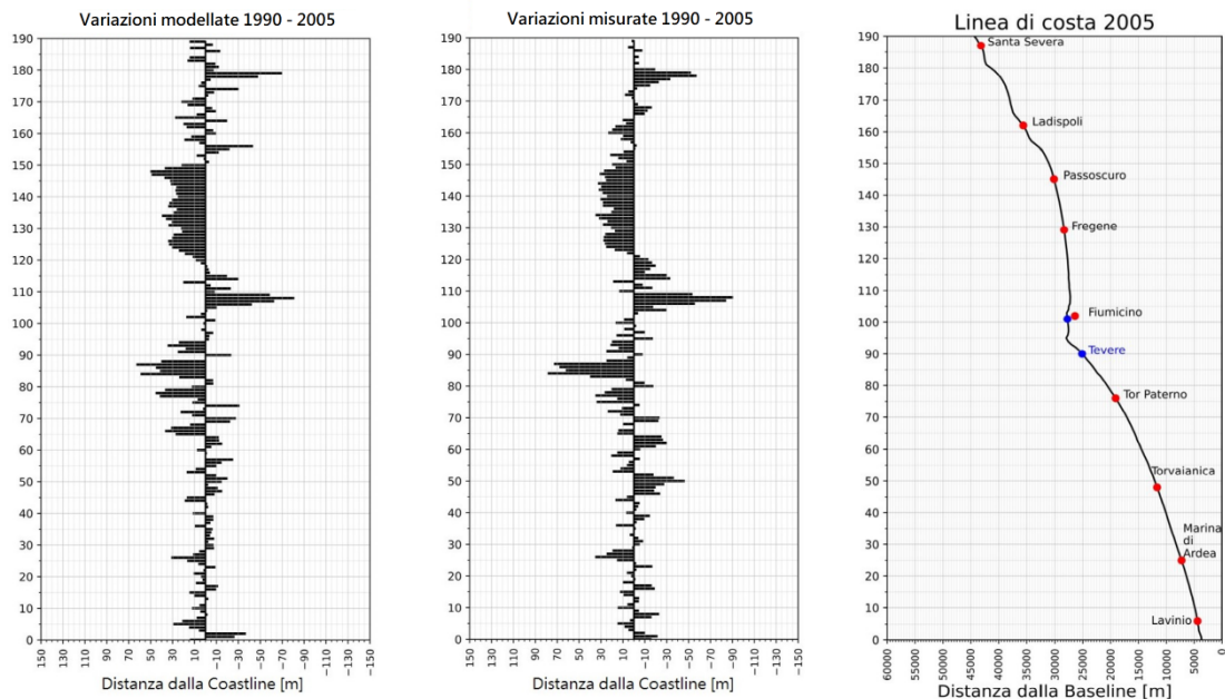
Fig. 94 Variazioni della linea di costa riprodotte con il modello LITPACK (a sinistra) e osservate da foto aeree e immagini satellitari (al centro) nel periodo compreso tra il 1990 e il 2005. Linea di costa rappresentativa dell'unità fisiografica Capo Linaro - Capo d'Anzio in cui vengono riportate alcuni comuni costieri in rosso e la foce dei fiumi in blu (a destra)
