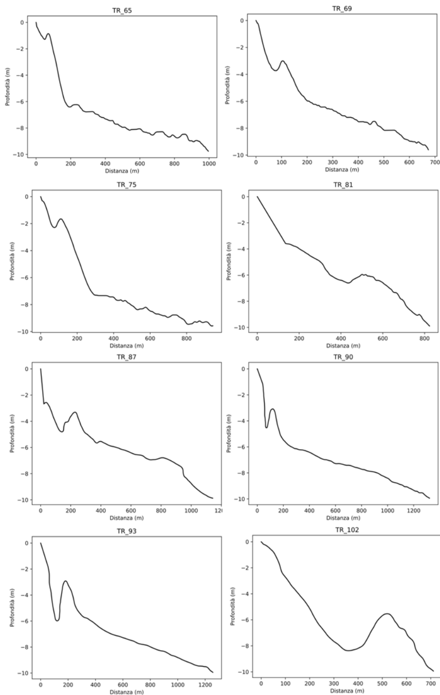
Figura 79 alcuni profili batimetrici della zona centrale
