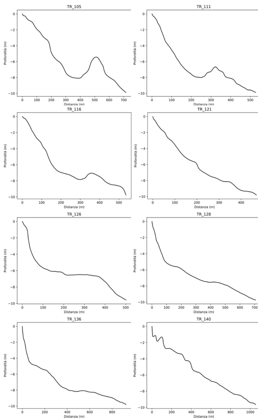
Figura 80 alcuni profili batimetrici della zona a sud
