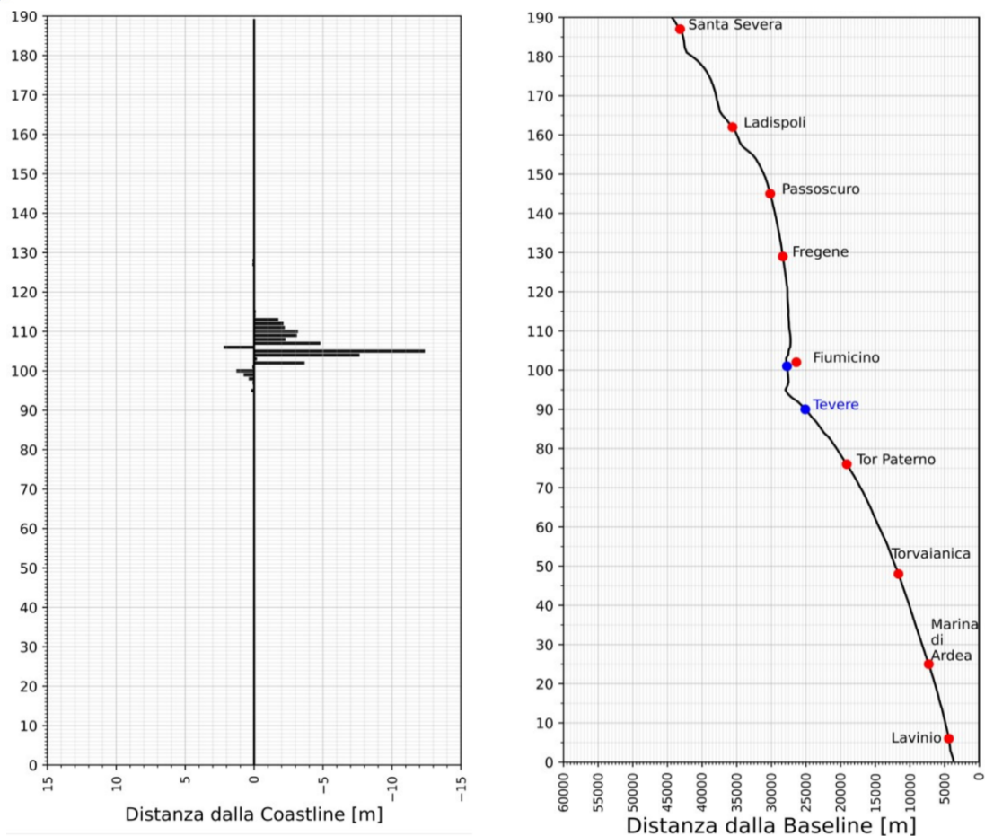
Fig. 96 Variazioni della linea di riva dovute alla presenza dell'opera (1° Lotto Funzionale) ottenute sottraendo i cambiamenti prodotti in sua assenza (a sinistra). Linea di costa rappresentativa dell'unità fisiografica Capo Linaro - Capo d'Anzio in cui vengono riportate alcuni comuni costieri in rosso e la foce dei fiumi in blu (a destra)
