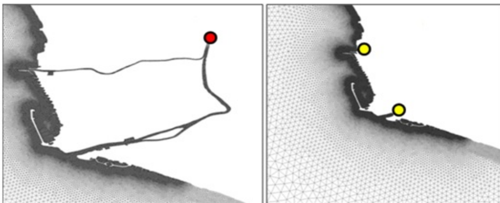
Fig.51 configurazioni utilizzate nel modello Shyft per riprodurre l'input fluviale del fiume Tevere: a sinistra la configurazione RCO a destra quella CO
