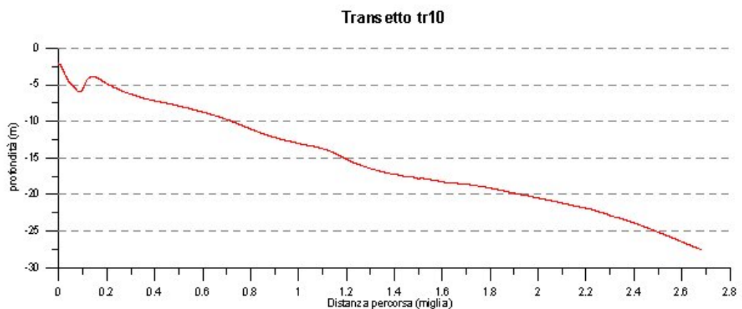
Fig. 86 Profilo batimetrico relativo al transetto "tr10"
