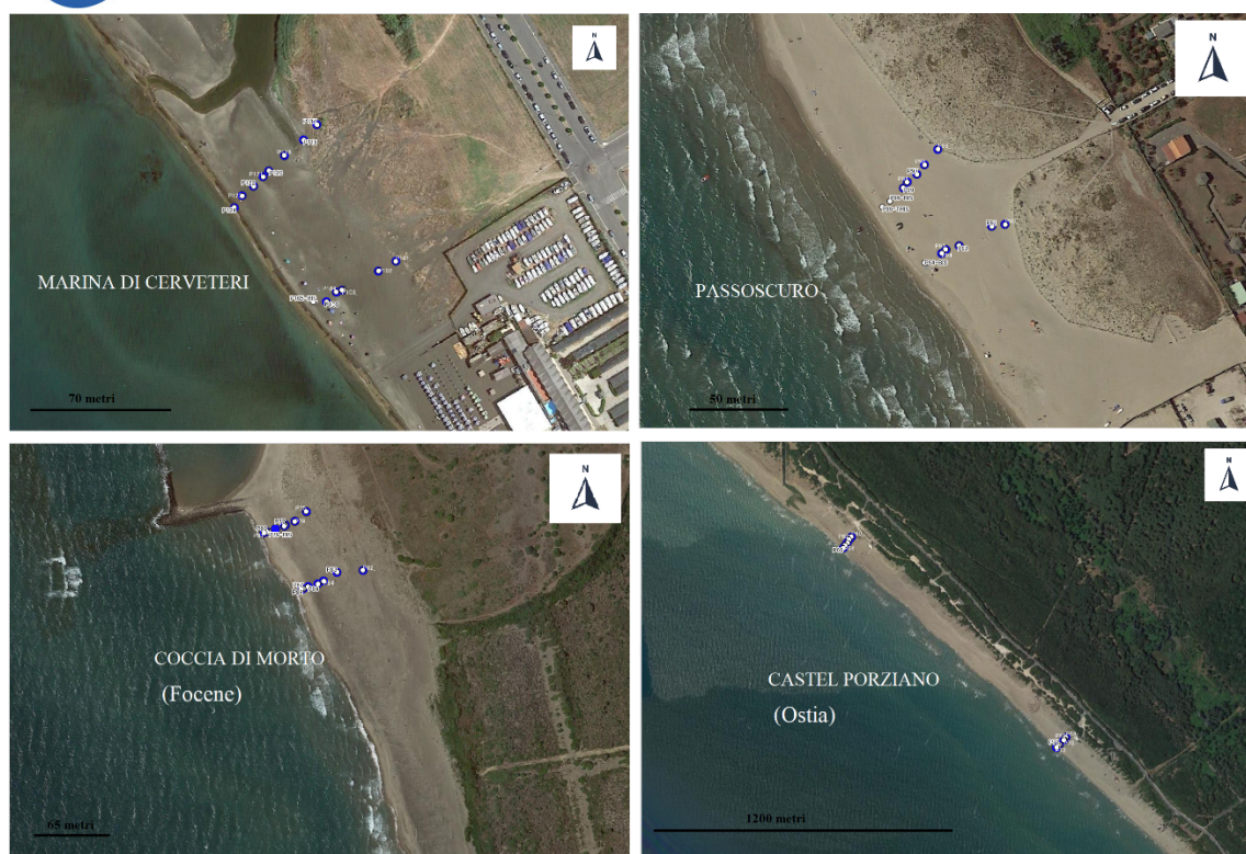
Fig. 38 Ubicazione dei transetti di misura morfologica della spiaggia emersa.
