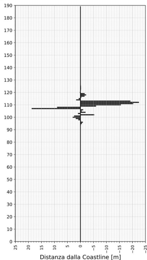
Fig. 97 Variazioni della linea di riva dovute alla presenza dell'opera (Configurazione completa) ottenute sottraendo i cambiamenti prodotti in sua assenza (a sinistra). Linea di costa rappresentativa dell'unità fisiografica Capo Linaro - Capo d'Anzio in cui vengono riportate alcuni comuni costieri in rosso e la foce dei fiumi in blu (a destra)
