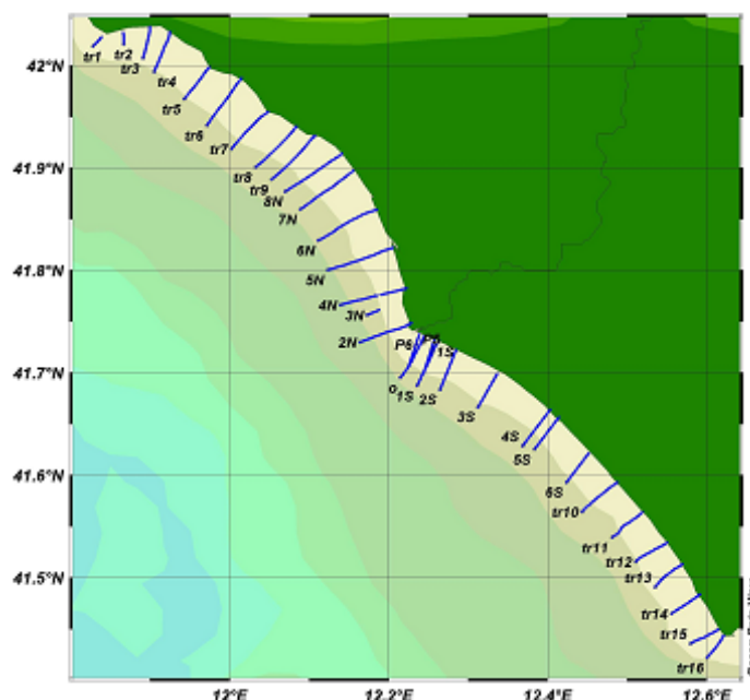
Fig. 81 Rappresentazione dei transetti batimetrici acquisiti tra il 2005 e il 2006
