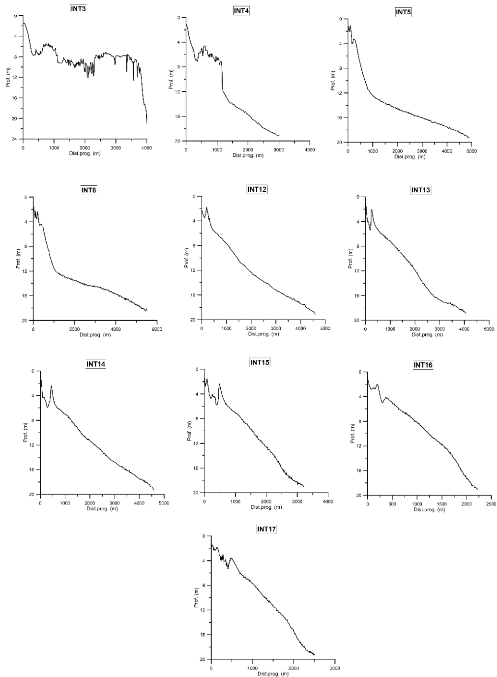
Fig. 30 Profili morfologici acquisiti durante la campagna integrativa 2021.
