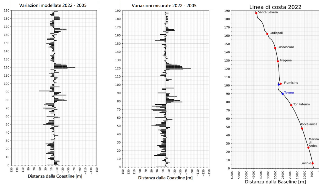
Fig. 95 Variazioni della linea di costa riprodotte con il modello LITPACK (a sinistra) e osservate da foto aeree e immagini satellitari (al centro) nel periodo compreso tra il 2005 e il 2022. Linea di costa rappresentativa dell'unità fisiografica Capo Linaro - Capo d'Anzio in cui vengono riportate alcuni comuni costieri in rosso e la foce dei fiumi in blu (a destra)
