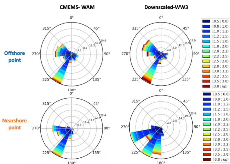
Figura 63 diagrammi polari in due punti significativi (offshore e nearshore) di moto ondoso per il modello d'onda di Fiumicino basato su WW3 e per il modello di CMEMS basato su WAM
