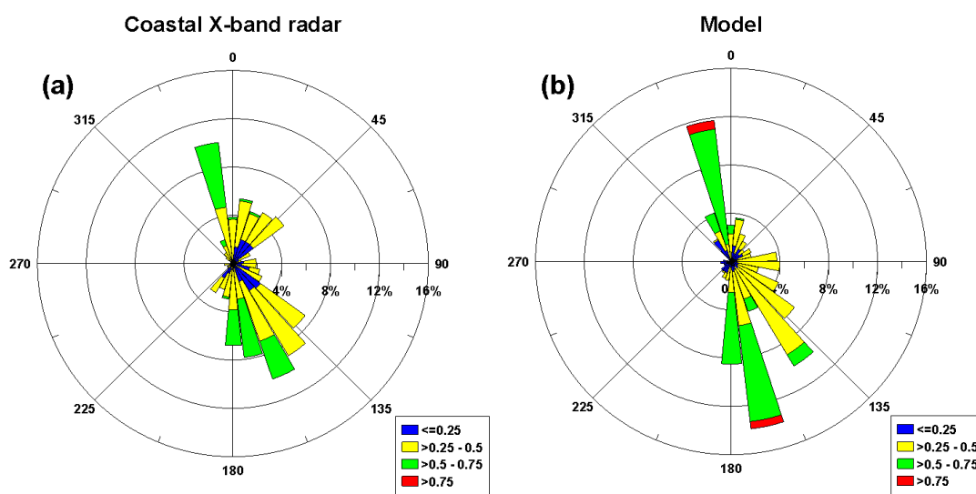
Fig. 59 Diagrammi polari del campo di velocità osservato (a) e modellato (b) ottenuto attraverso la media dell'intero dominio del radar.
