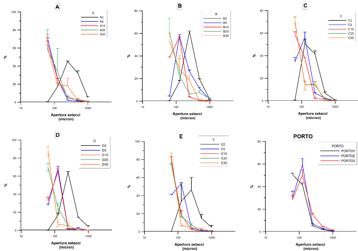
Fig. 37 Curve di frequenza relativa della frazione sabbiosa dei campioni analizzati.
