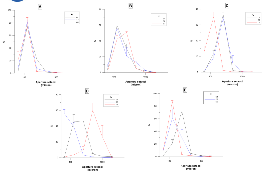
Fig. 33 Curve di frequenza relativa dei campioni prelevati durante la stagione estiva (agosto 2020)
