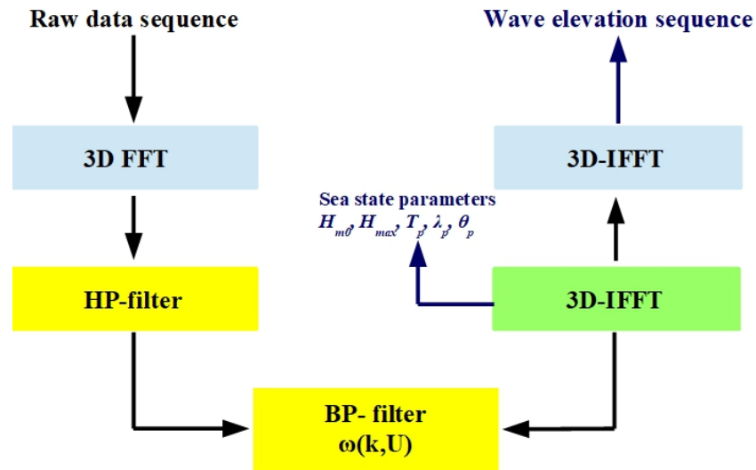
Fig.5 Diagramma a blocchi che descrive il processing delle immagini radar. Il dettaglio dei parametri di acquisizione del radar sono riportati in Tabella 1.
