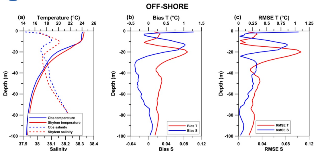
Fig. 56 Validazione del modello con i dati CTD della zona off-shore in termini di temperatura e salinità media (a). Vengono mostrate inoltre i profili di bias (b) e RMSE (c)
