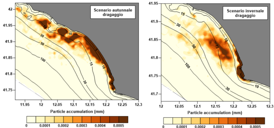
Fig. 68 zone di accumulo del sedimento fine proveniente dalle attività di dragaggio nella condizione autunnale (a sinistra) ed invernale (a destra)
