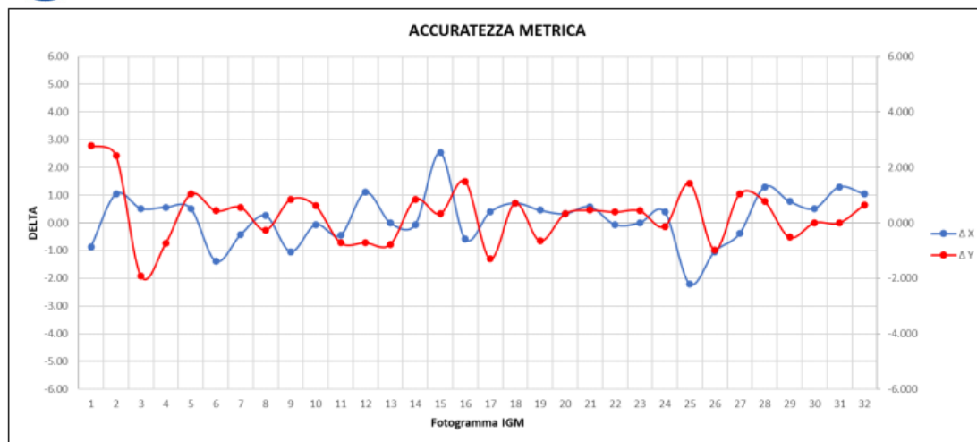
Fig.73 Confronto della RMSE in X e in Y tra tutti i fotogrammi ortorettificati
