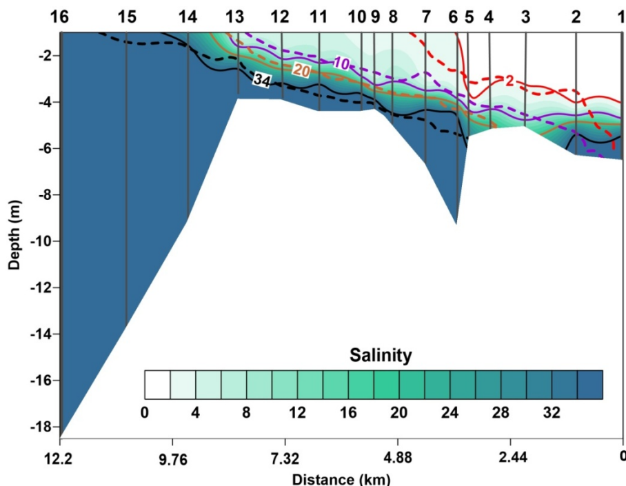
Fig. 61 Sezione trasversale di salinità lungo il ramo di Fiumara Grande. I contorni continui rappresentano le osservazioni, mentre le linee tratteggiate indicano i valori modellati
